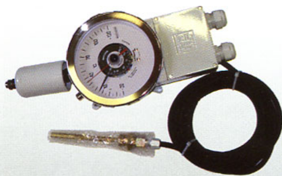
Termometr czterokontaktowy MSRT 150
