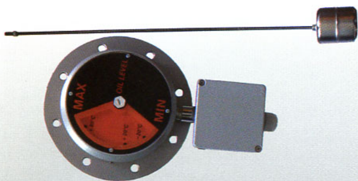
Magnetyczny wskaźnik poziomu oleju OL 220
