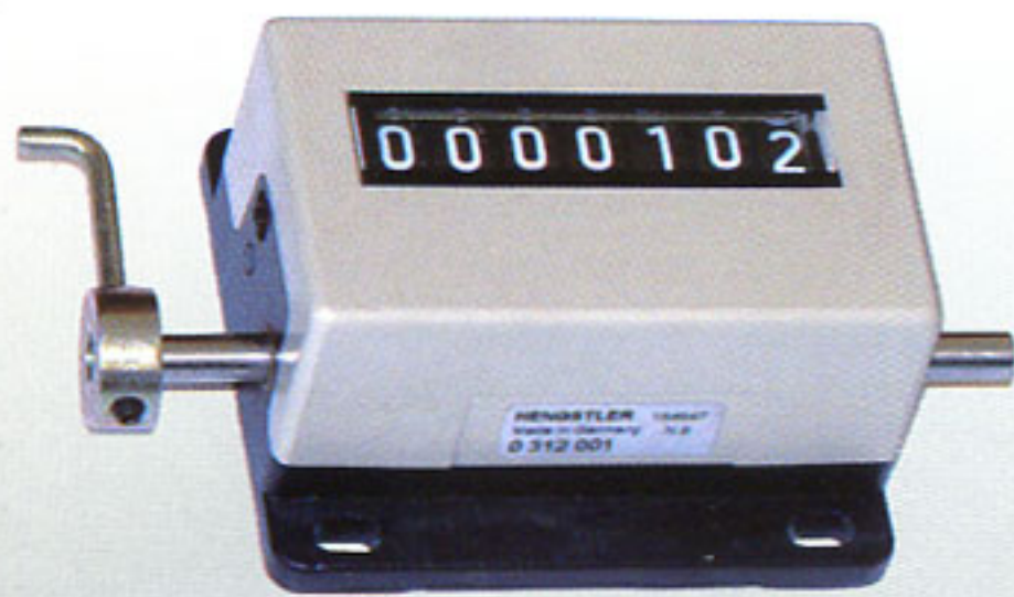
Licznik napędu
