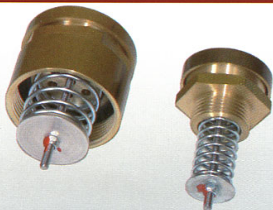
Zawory do transformatorów hermetycznych 1 i 2 cale
