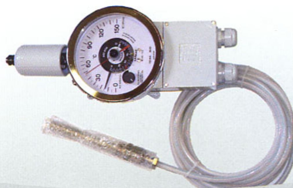
Termometr czterokontaktowy MSRT 150 W
